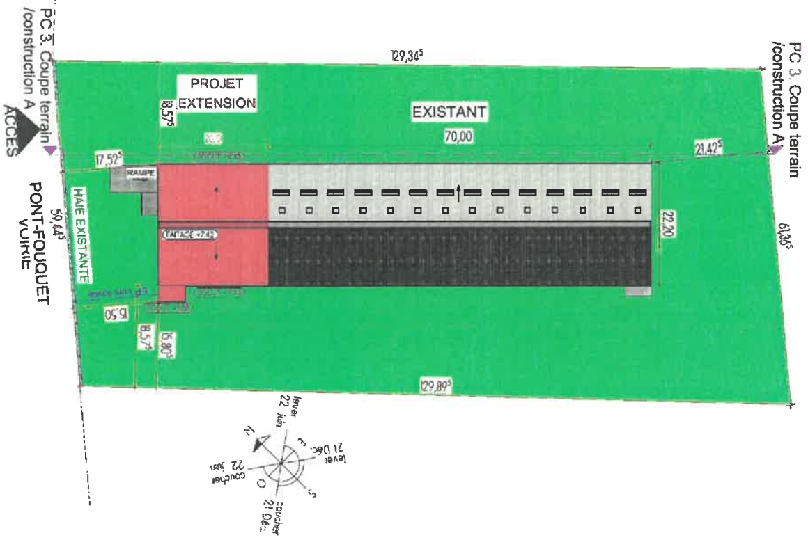
PC2. PLAN MASSE 1/500
